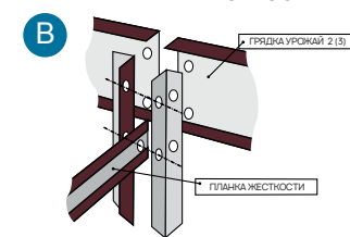
МОНТАЖ ПЛАНКИ ЖЕСТКОСТИ
