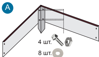
СОЕДИНЕНИЕ ПАНЕЛЕЙ ВСТЫК
