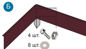
МОНТАЖ ПЛАНКИ ЖЕСТКОСТИ
