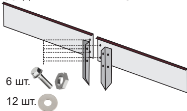
СОЕДИНЕНИЕ ПАНЕЛЕЙ ВСТЫК
